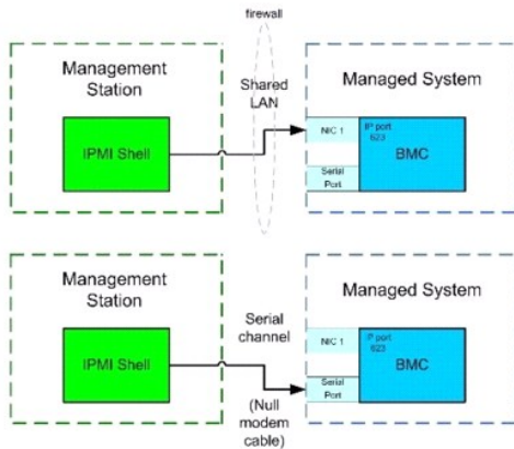
图 3-2. IPMI Shell 图
